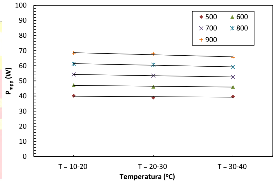
Figura 11: P_{mpp} para el módulo A para los intervalos de temperatura estudiados en la figura 9. Los valores de P_{mpp} han sido calculados con las ecuaciones lineales obtenidos en dicha figura a distintos niveles de DNI con el objetivo de estimar la influencia de la temperatura. En concreto para niveles de DNI de 500, 600, 700, 800, y 900 W/m^2 .
