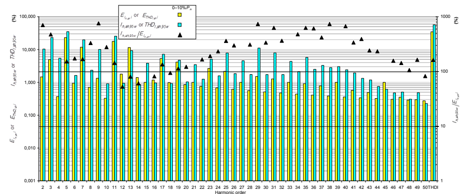
Figura 4. Resultado particular de medidas armónicas para índices de tiempo corto ( I_{h,sh,95w} , THDI_{sh,95w} ) frente a los objetivos correspondientes de emisión de corriente armónica en la planta CPV de 800 kWp en el intervalo de potencia activa (0-10%).
