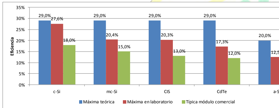
Figura 2.3: Eficiencias máximas y típicas alcanzadas por módulos fotovoltaicos de las diferentes tecnologías.
