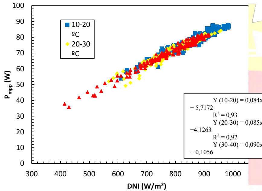
Figura 9: P_{mpp} versus DNI para el módulo A clasificado por temperaturas. Todas las medidas son filtradas para AM \leq 2 para minimizar efectos espectrales.
