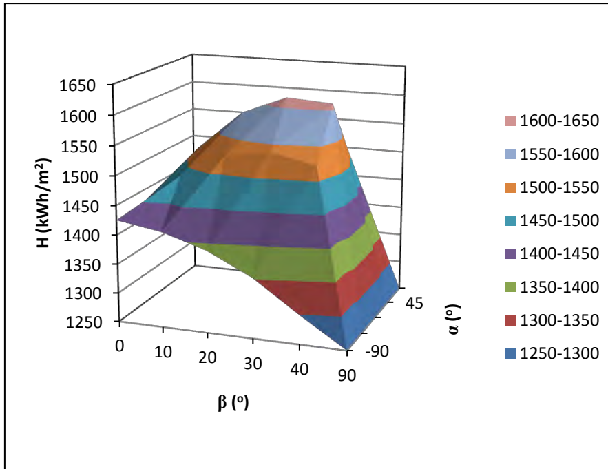
Figura 3.1: Distribución de la irradiación anual en kWh/m 2 para León, España.
