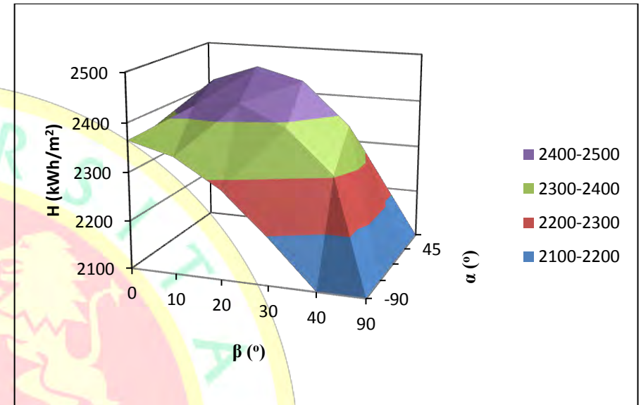
Figura 3.4: Distribución de la irradiación anual en kWh/m 2 para La Meca, Arabia Saudita.
