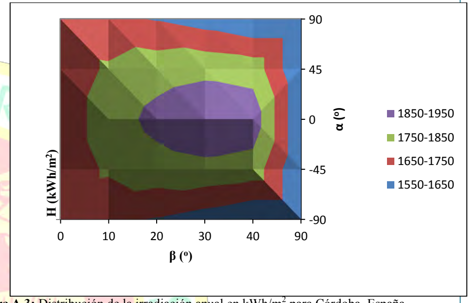
Figura A.3: Distribución de la irradiación anual en kWh/m 2 para Córdoba, España.
