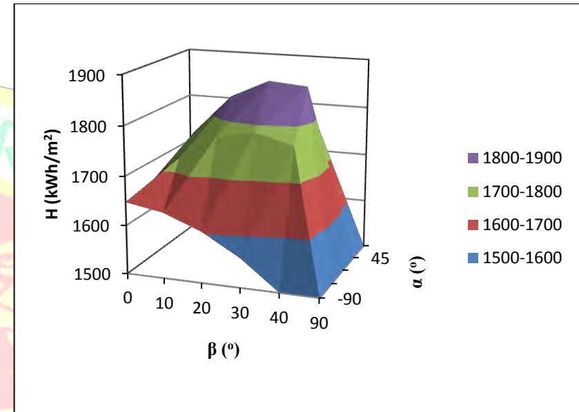
Figura 3.2: Distribución de la irradiación anual en kWh/m 2 para Madrid, España.
