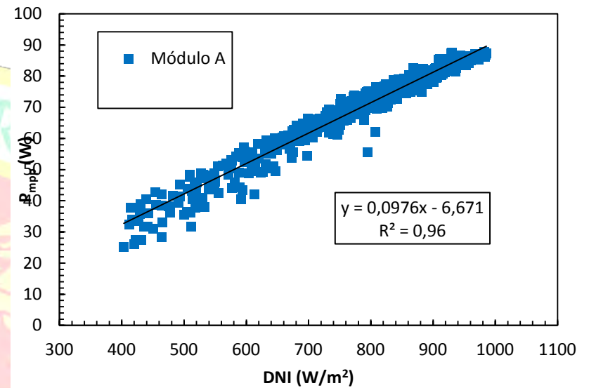
Figura 4: P_{mpp} versus DNI para el módulo A para radiaciones mayores de 400 W/m^2 .
