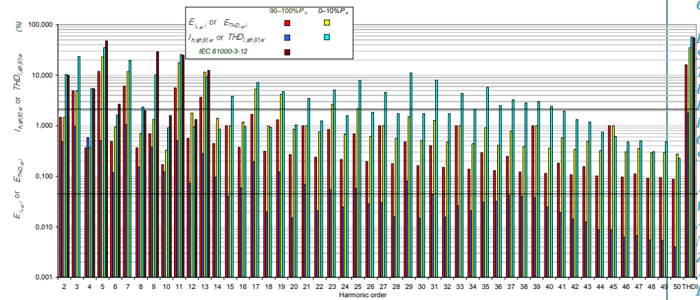
Figura 3. Resultado de medidas armónicas para índices de tiempo corto ( I_{h,sh,95w} , THDI_{sh,95w} ) frente a los objetivos correspondientes de emisión de corriente armónica en la planta CPV de 800 kWp en dos intervalos de potencia activa (0-10% y 90-100%); objetivos para cualquier inversor CPV individual de esta unidad de generación distribuida CPV .
