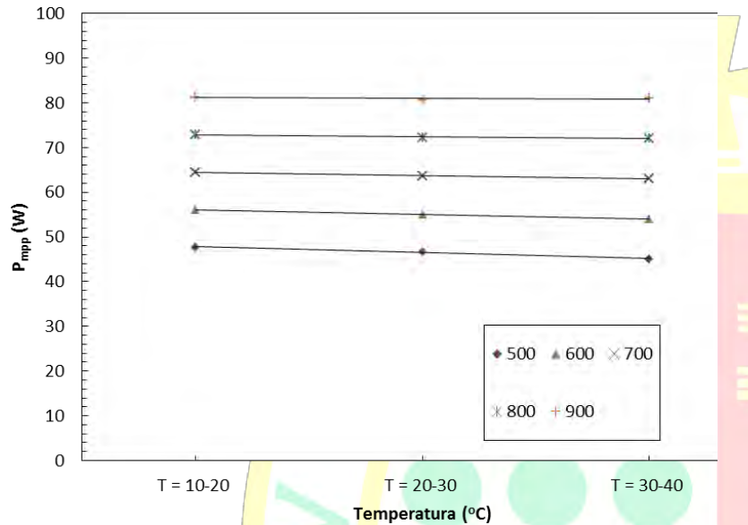
Figura 11: P_{mpp} para el módulo A para los intervalos de temperatura estudiados en la figura 9. Los valores de P_{mpp} han sido calculados con las ecuaciones lineales obtenidos en dicha figura a distintos niveles de DNI con el objetivo de estimar la influencia de la temperatura. En concreto para niveles de DNI de 500, 600, 700, 800, y 900 W/m^2 .
