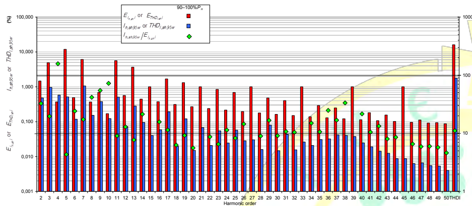
Figura 5. Resultado particular de medidas armónicas para índices de tiempo corto ( I_{h,sh,95w} , THDI_{sh,95w} ) frente a los objetivos correspondientes de emisión de corriente armónica en la planta CPV de 800 kWp en el intervalo de potencia activa (90–100%).
