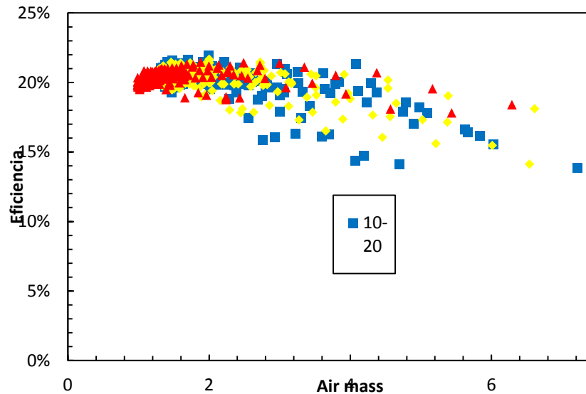
Figura 7: Eficiencia versus AM para el módulo A clasificado por intervalos de temperatura.
