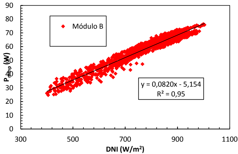
Figura 5: P_{mpp} versus DNI para el módulo A para radiaciones mayores de 400 W/m^2 .
