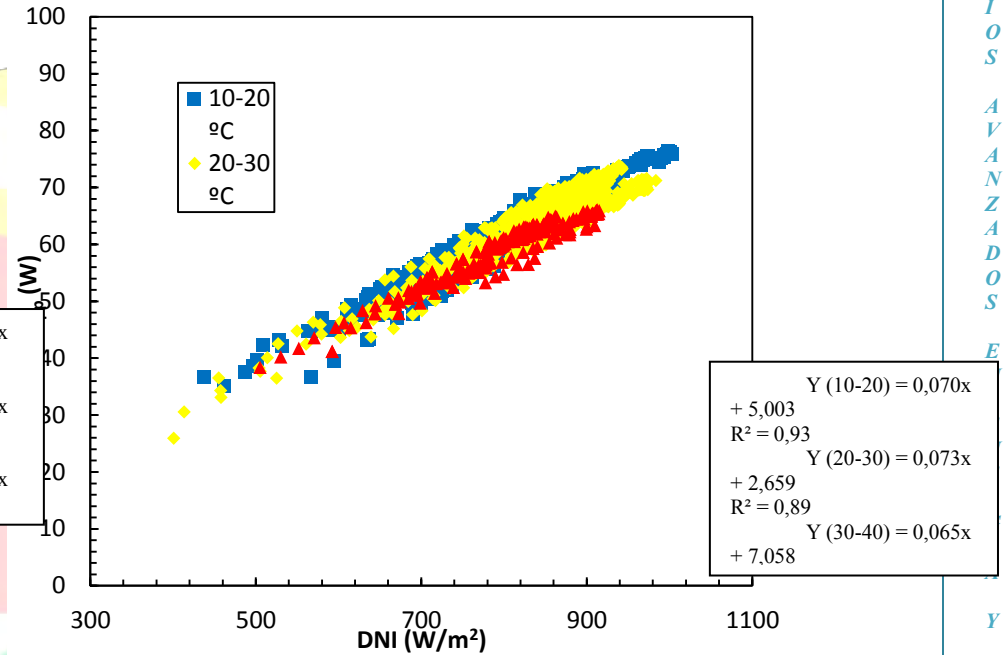
Figura 10: P_{mpp} versus DNI para el módulo B clasificado por temperaturas. Todas las medidas son filtradas para AM \leq 2 para minimizar efectos espectrales.
