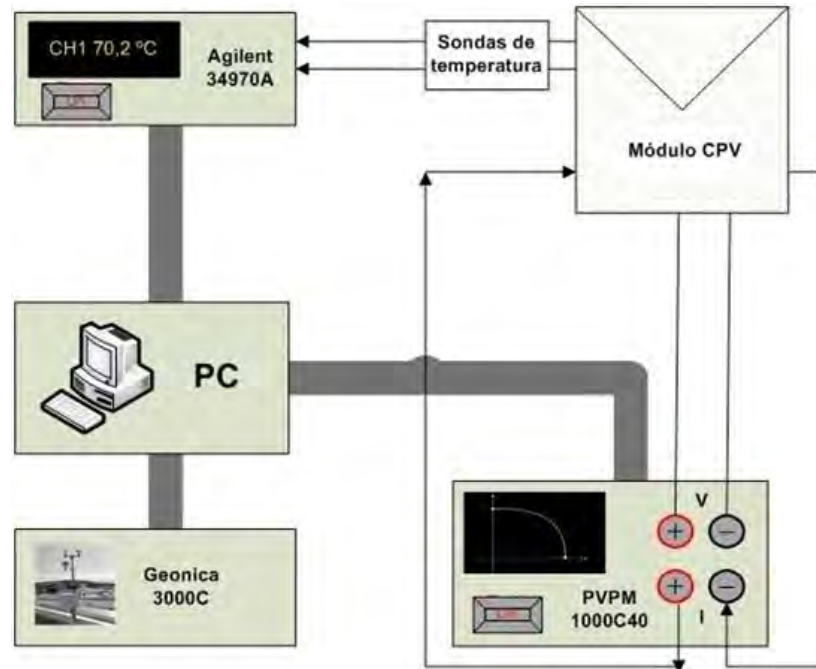
Figura 2: Esquema del sistema de medidas para la medición de los módulos CPV bajo estudio
