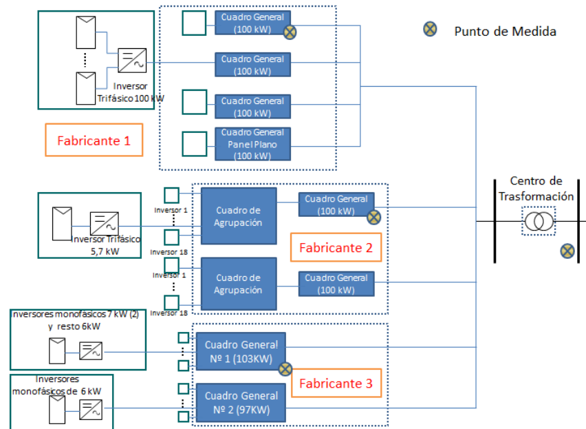
Figura 2 . Puntos de medida de la planta CPV y distribución de la planta.
