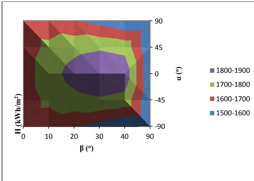
Figura A.2: Distribución de la irradiación anual en kWh/m 2 para Madrid, España.
