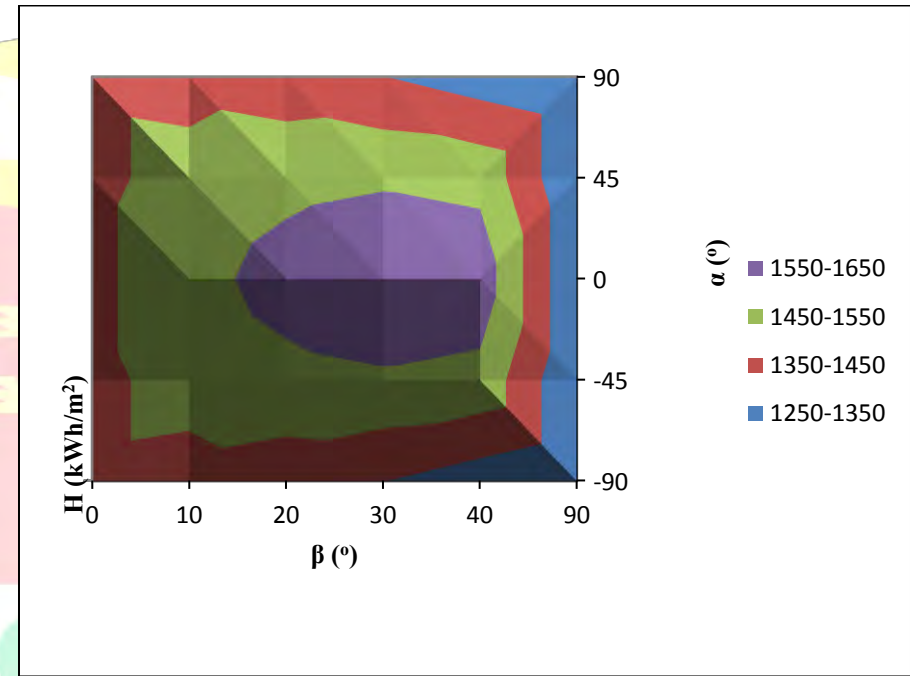
Figura A.1: Distribución de la irradiación anual en kWh/m 2 para León, España.
