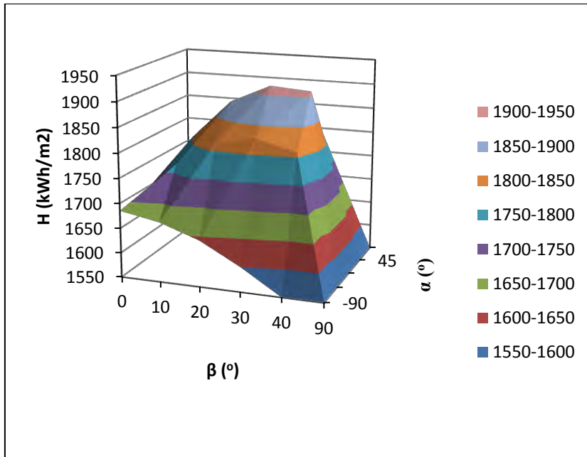
Figura 3.3: Distribución de la irradiación anual en kWh/m 2 para Córdoba, España.
