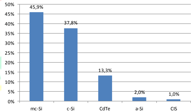
Figura 2.2: Porcentaje de la potencia fotovoltaica instalada a nivel mundial por tipo de tecnología.
