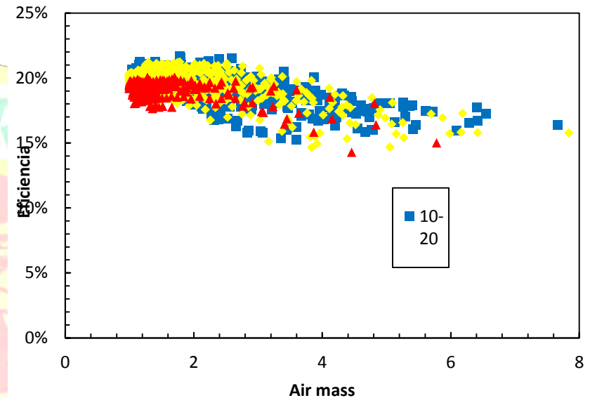
Figura 8: Eficiencia versus AM para el módulo B clasificado por intervalos de temperatura.
